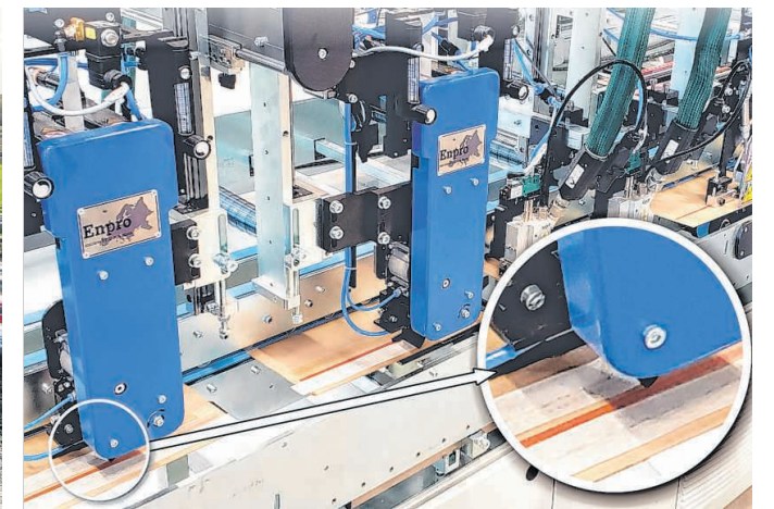
Enpro-Aggregate im Einsatz: Trennpapierstreifen (weiß) und Aufreißfäden (rot) werden auf Kartonzuschnitte appliziert.
